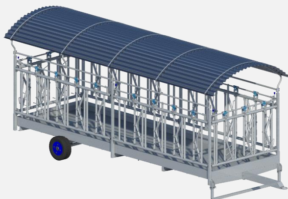
Pašne jaslji – KLASIČNE ALI Z ZAPORNICAMI NA KOLESIH (14 in 22 glav)
